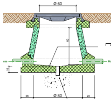
Abbildung 10 Kabelkanalisation: Kontrollschacht
