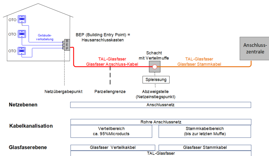
Abbildung 16 TAL-Glasfasern: Schema
