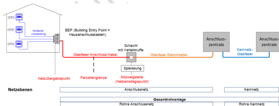
Abbildung 14 Kabelkanalisation: Schema
