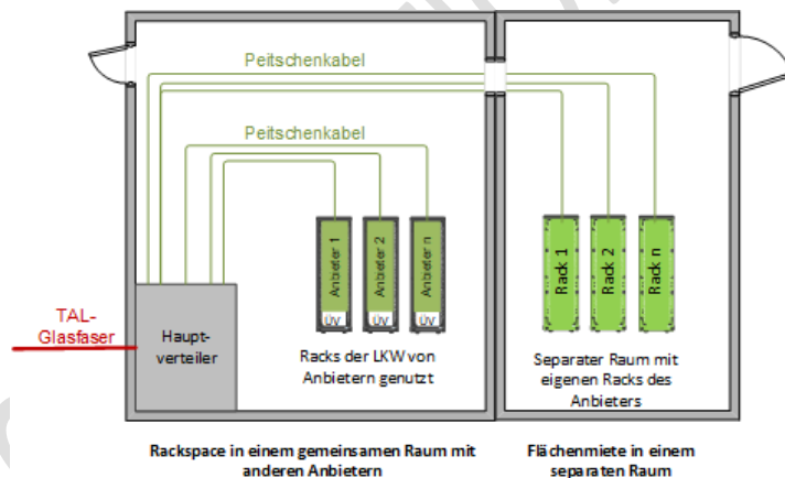
Abbildung 13 Anschlussszentrale: Rackspace Shared Room (links) und Private Room (rechts)
