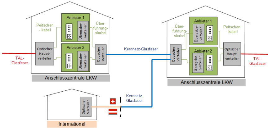
Abbildung 15 Kernnetz Glasfasern: Schema
