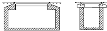
Abbildung 7 Kabelkanalisation: Kleineinstiegschacht
