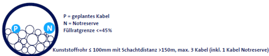
Abbildung 23 Kabelkanalisation: Frei verfügbare Kapazitäten bzw. Reserven - Kunststoffrohre
